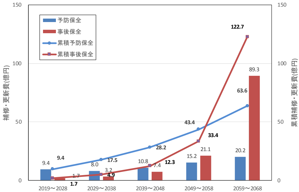
図-2 今後50年の維持管理コストの比較
